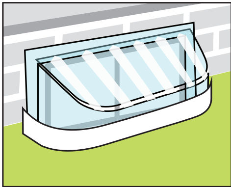
Instalar poços de luz (window wells) 10 a 15 cm acima do solo e as respectivas coberturas (onde permitido pelas normas de segurança contra incêndios). Vedar vazamentos em janelas e fundações e vedar todos os poços de luz. 10 a 15 cm (4 a 6")
